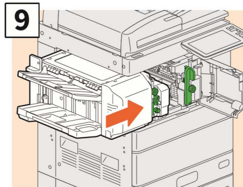
小心复位整理器。
