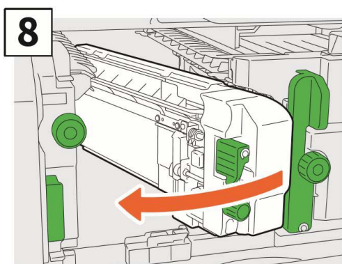
复位打孔单元。
